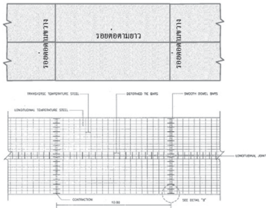
รูปที่ 6-47 (ก) แปลนถนนคอนกรีต ชนิดชั้นรองพื้นทางลูกรัง
