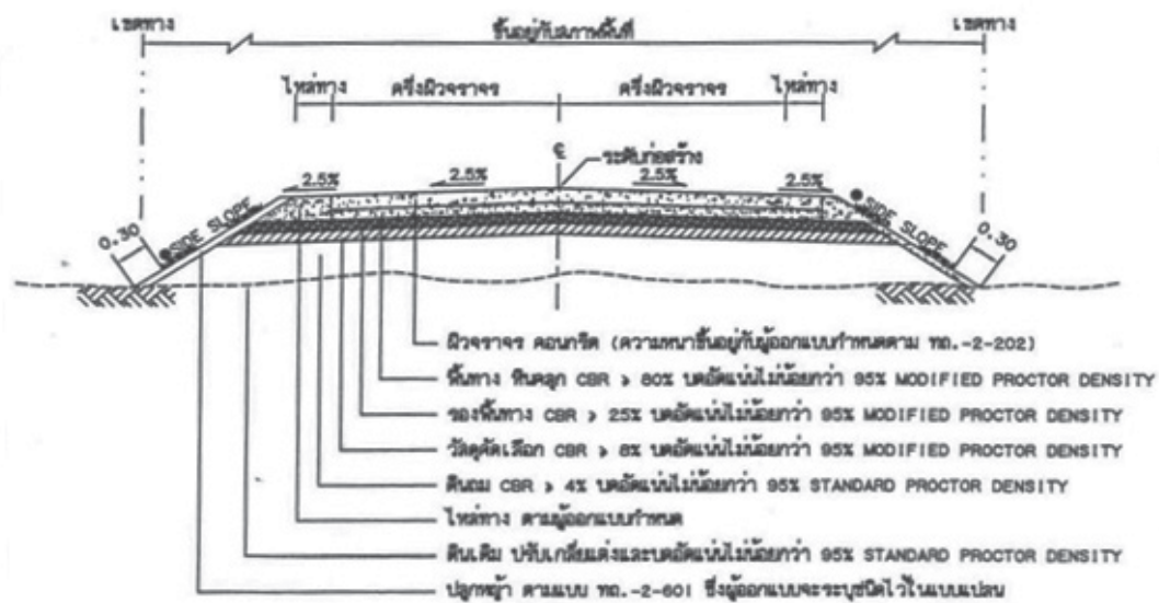
รูปที่ 6-47 (ข) รูปตัดถนนคอนกรีต ชนิดชั้นรองพื้นทางลูกรัง
